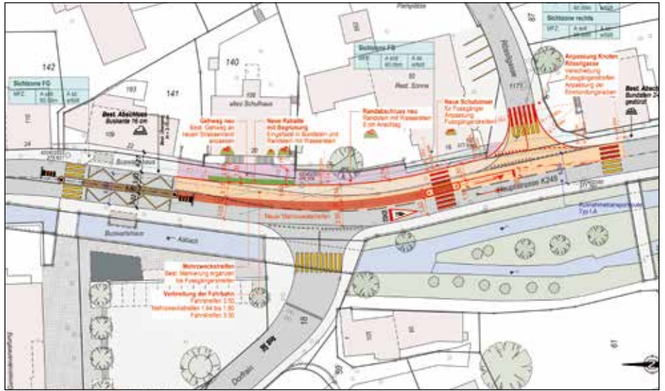
Sicherheitsstudie Variante 2: Der Antrag für das Projekt ist beim Kanton eingereicht, denn es handelt sich mit der Kantonsstrasse um das Entscheidungsgebiet des Kantons.
